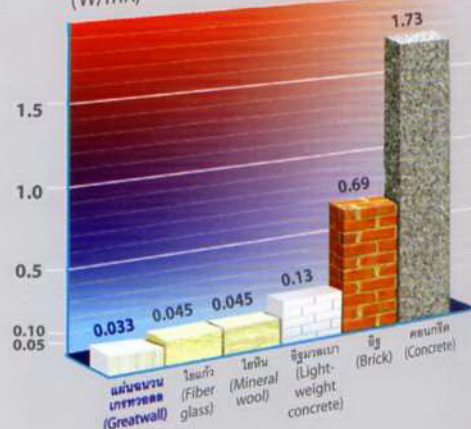
ค่าการนำความร้อน (Thermal Conductivity) (W/mK)
